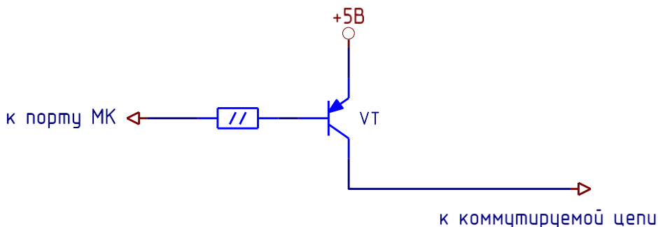
Рисунок 18 - Канал дискретного выхода
