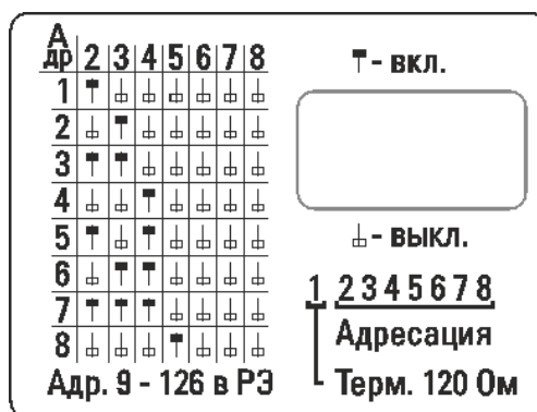
Рисунок 59 – Внешний вид DIP переключателя
