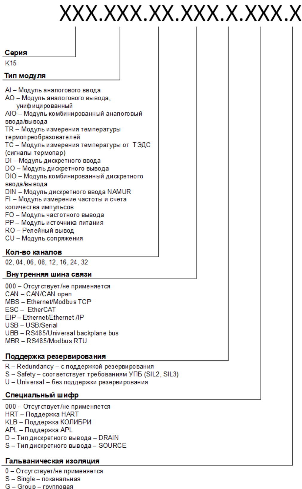
Рисунок 2 – Обозначение модулей ввода-вывода
