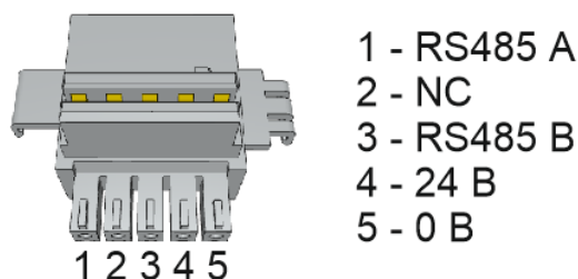
Рисунок 60 – Шинный соединитель T-BUS для модулей с интерфейсом связи RS
