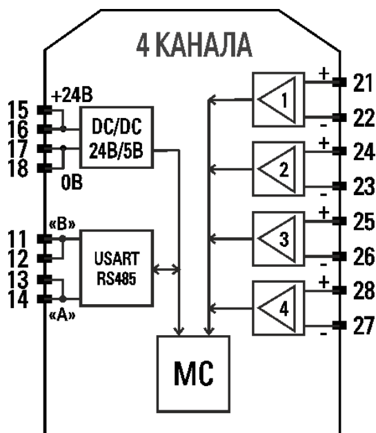
Рисунок 39 – Схема подключение модуля K15.AI4
