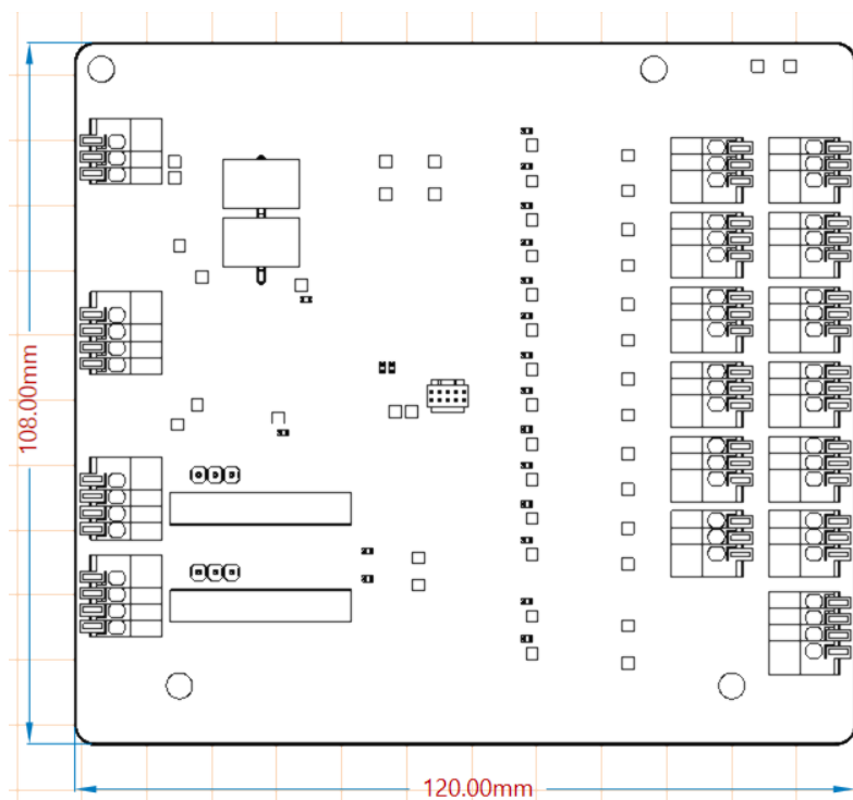
Рисунок 44 – Габаритные размеры модулей дискретного ввода K15.DI16.RS232
